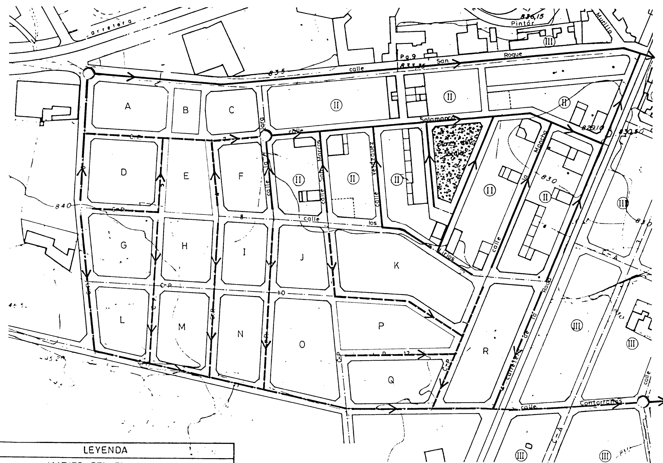
ESQUEMA RED DE SANEAMIENTO
