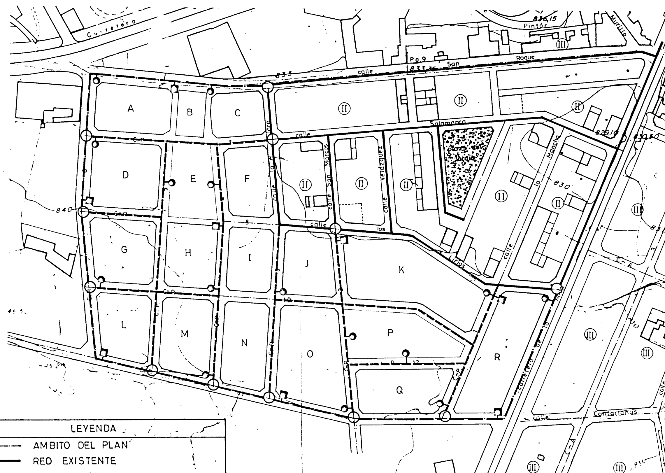
ESQUEMA RED DE AGUA POTABLE
