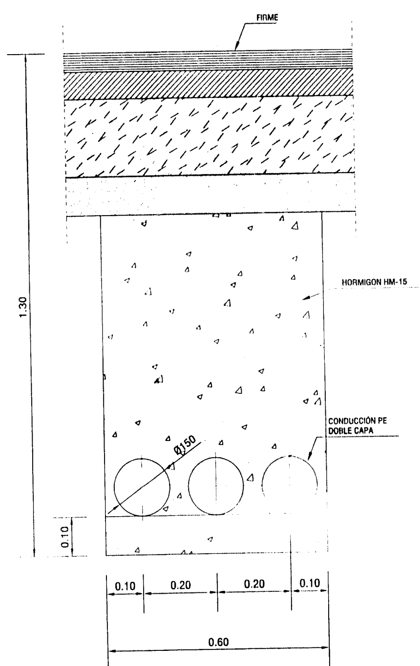
CANALIZACION PARA MEDIA O BAJA TENSION
