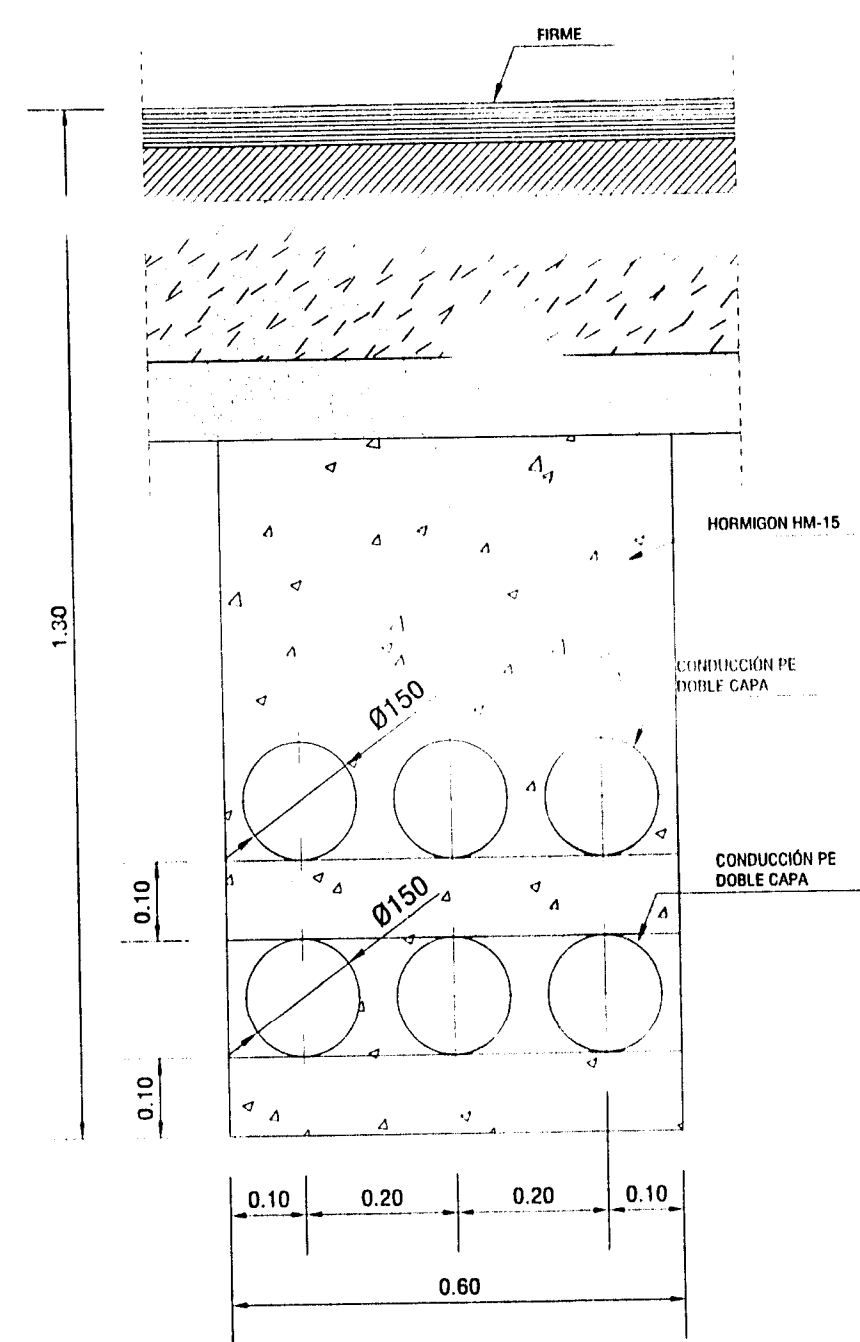
CANALIZACION PARA MEDIA Y BAJA TENSION
